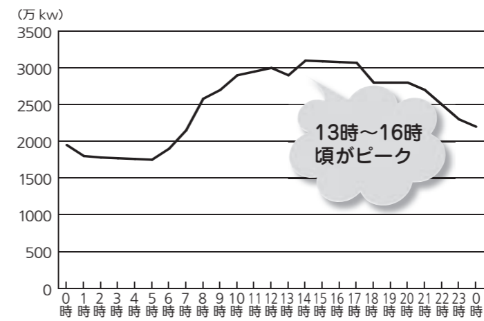
昨年の夏期最大電力発生日の電力使用量変化
